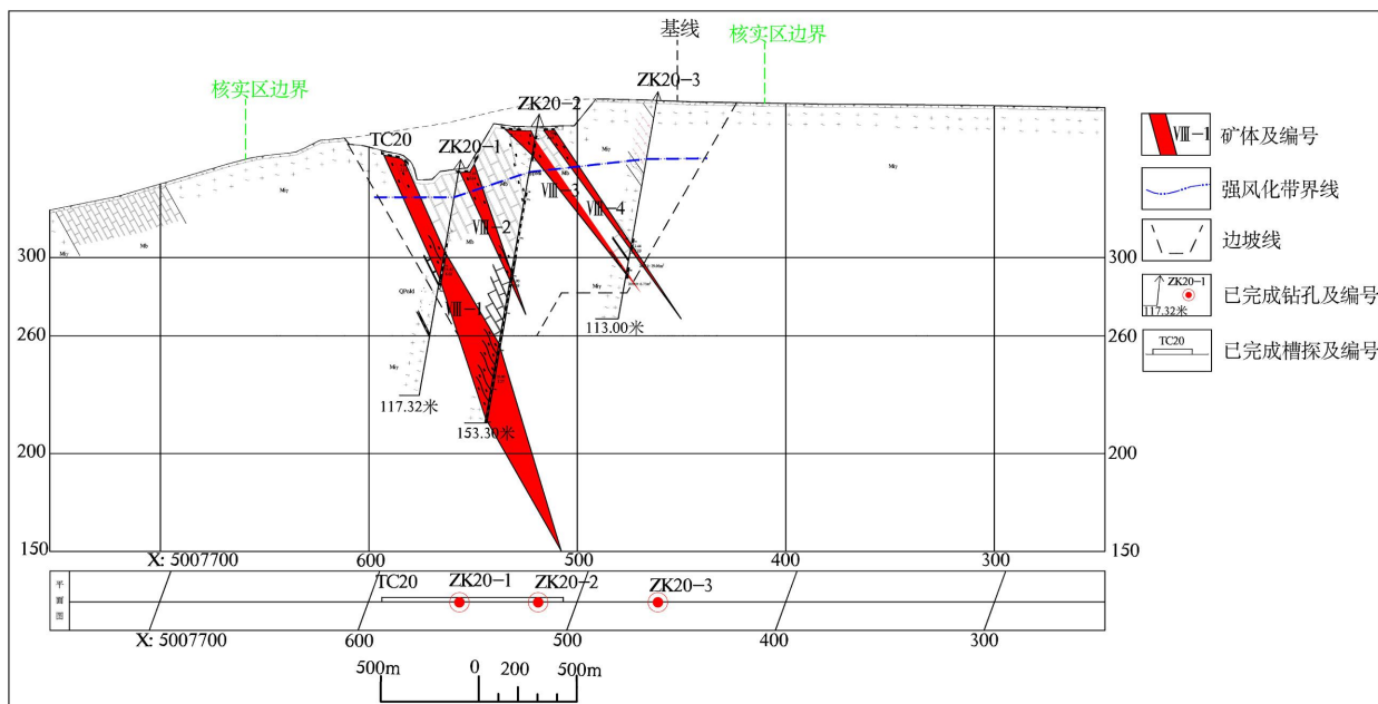
图1-6 友联一区20号勘探线剖面图
