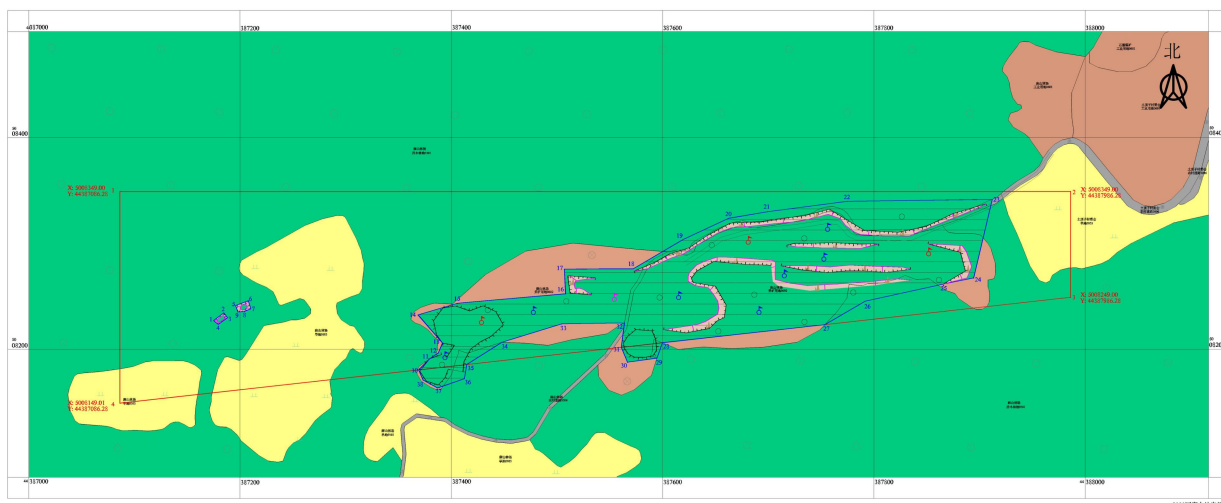
图 5-2 二区工程布置平面图
