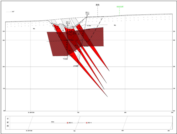
图 2-5 水文地质剖面图
