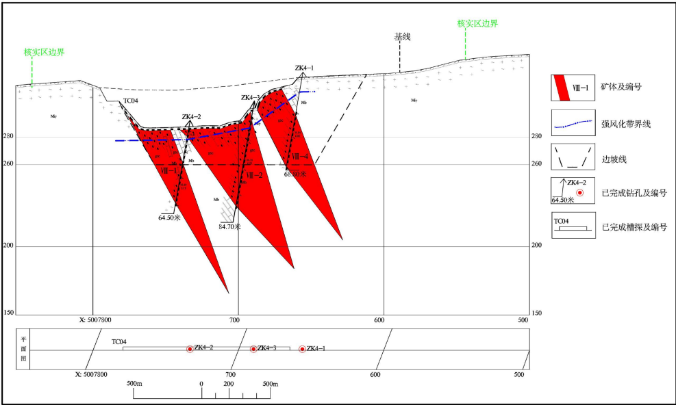
图 1-5 友联一区第 4 号勘探线剖面图
