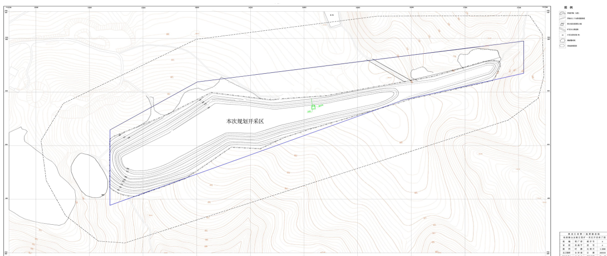
图 1-9 一区露天采场终了平面图
