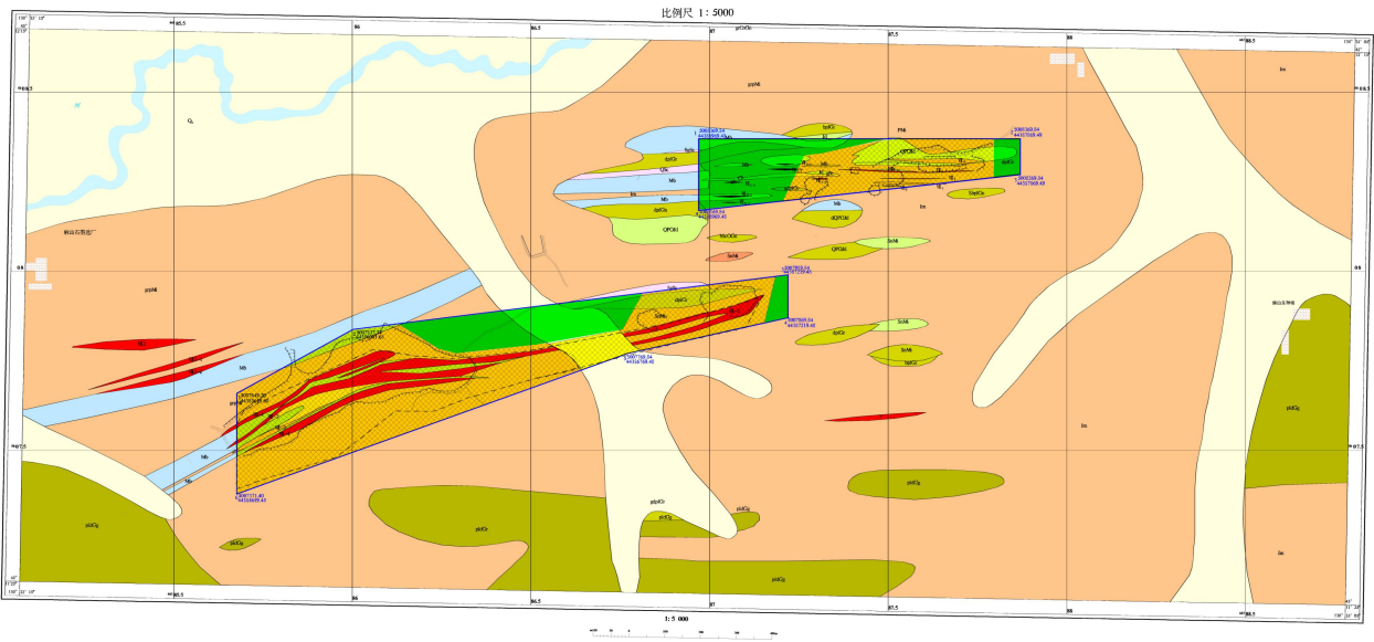
图 2-4 水文地质图
