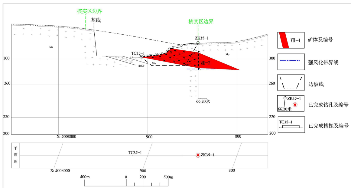
图1-7 友联一区35号勘探线剖面图
