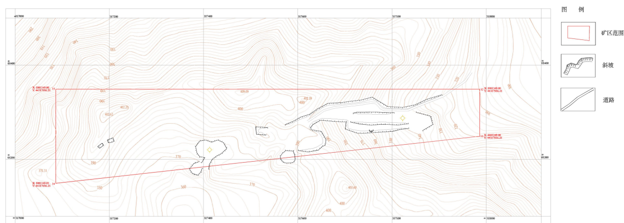
图 2-3 二区矿山地形地貌图
